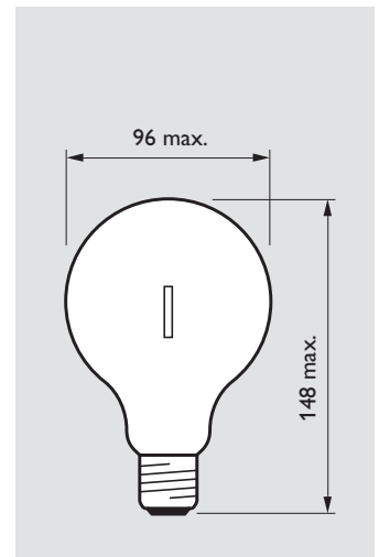
Globe E27
