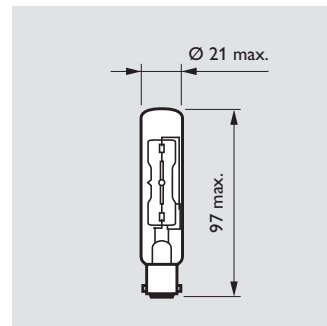
T20 B15d
