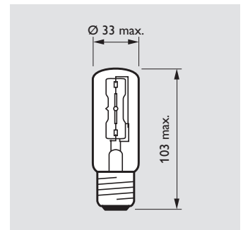
T32 E27
