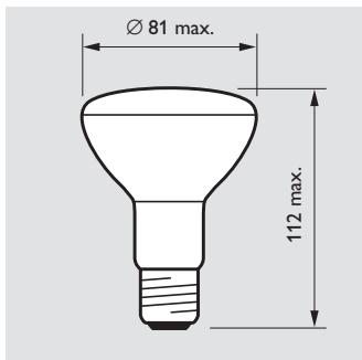
R80H E27
