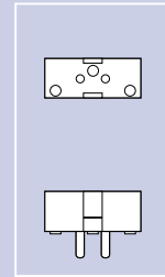
GX9.5 DIN: 49638 IEC: 7004-70A
